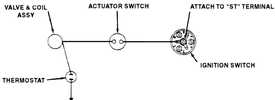
WIRING SCHEMATIC :
