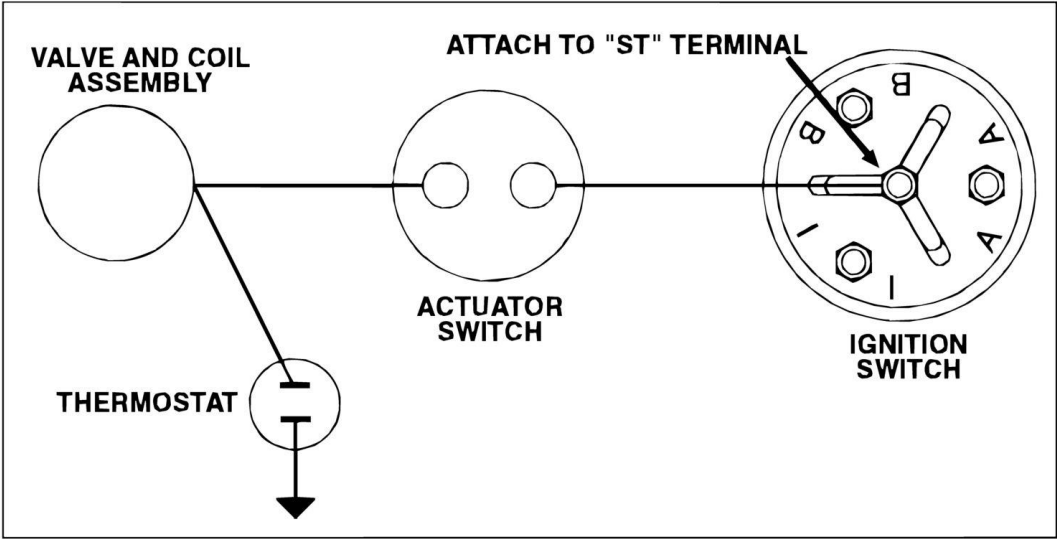
WIRING SCHEMATIC
