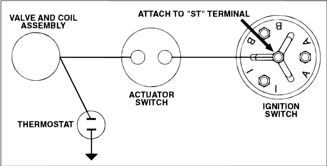
WIRING SCHEMATIC
